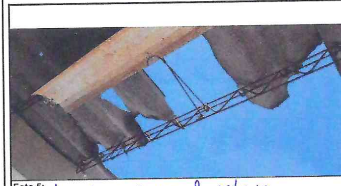
Foto 5: laminas en mal estado
